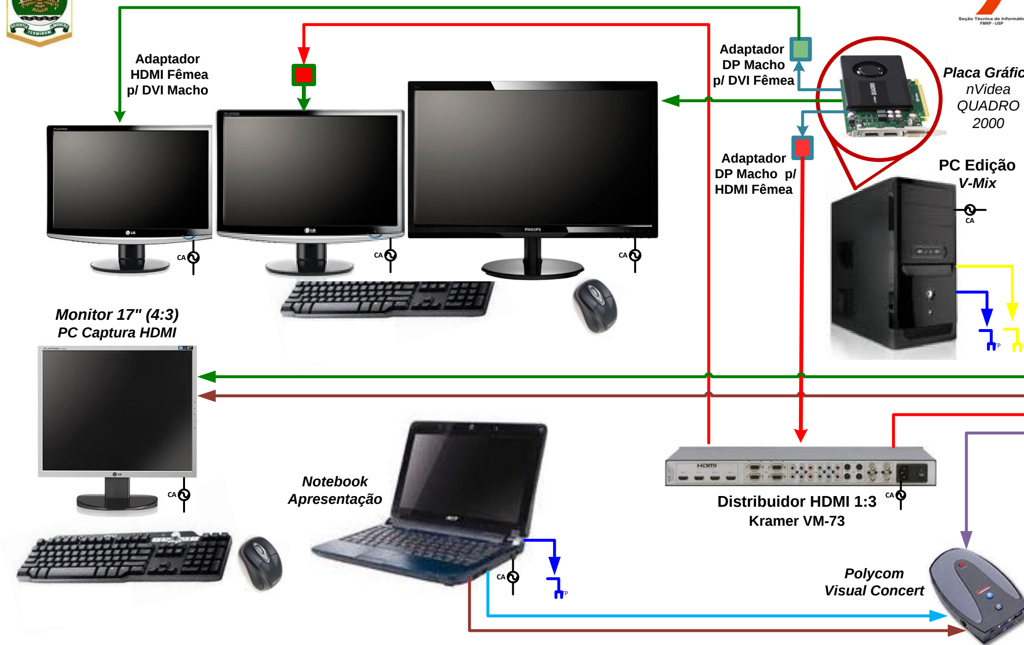
Figura 1: Projeto de Áudio & Vídeo – Sala de Controle do CPDig - FMRP/USP
