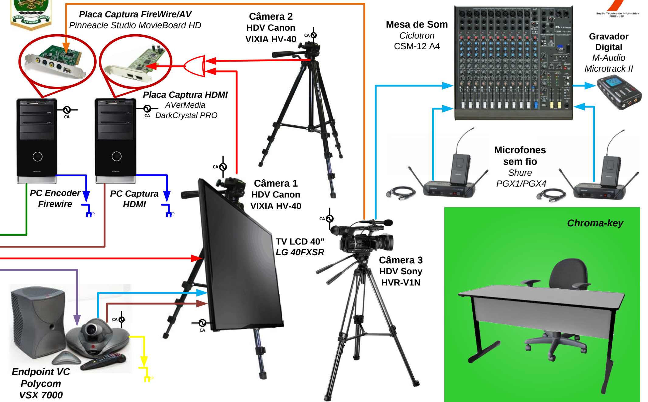
Figura 2: Projeto de Áudio & Vídeo - Estúdio do CPDig - FMRP/USP
