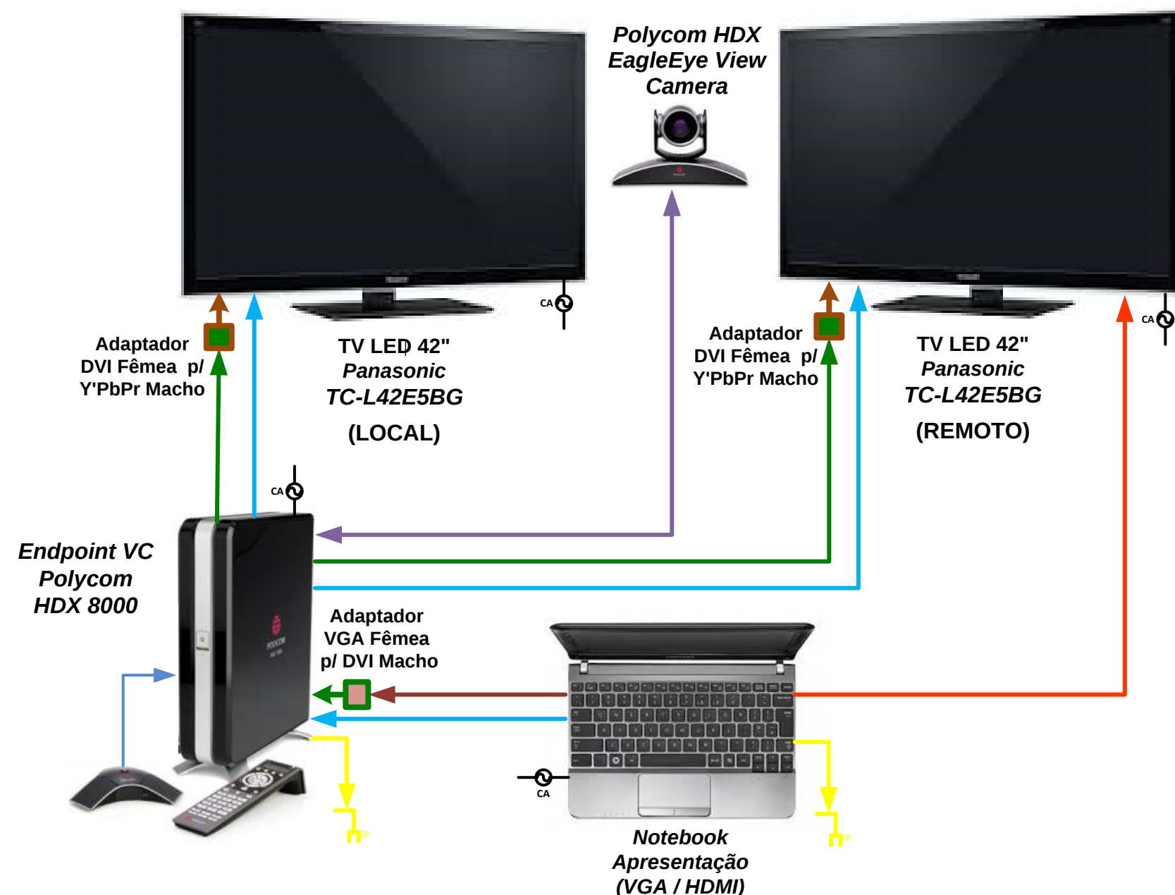
Figura 3: Projeto de Áudio & Vídeo – Sala de Reuniões do CPDig - FMRP/USP
