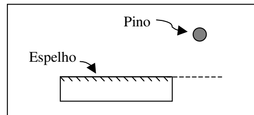
Figura 2.3 - Visão de topo do pino deslocado da frente para o lado do espelho plano.
