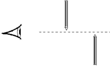
Figura 2.2 - Esquema do alinhamento dos lápis com o olho.
