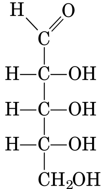
D-Ribose
