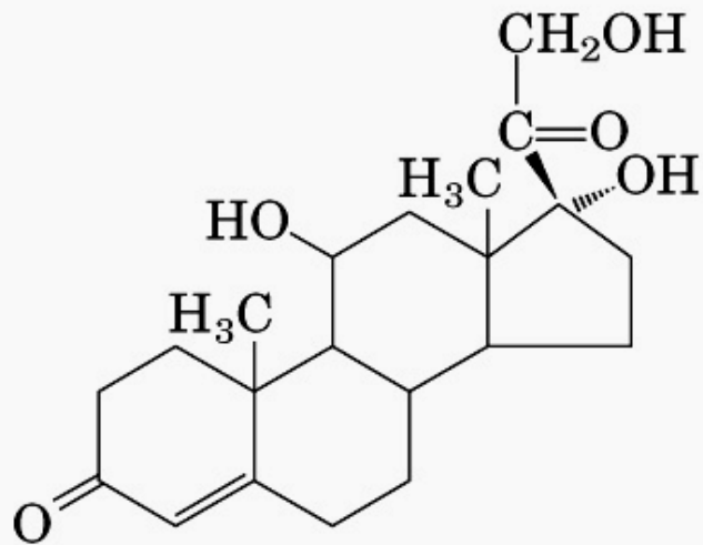
Cortisol
