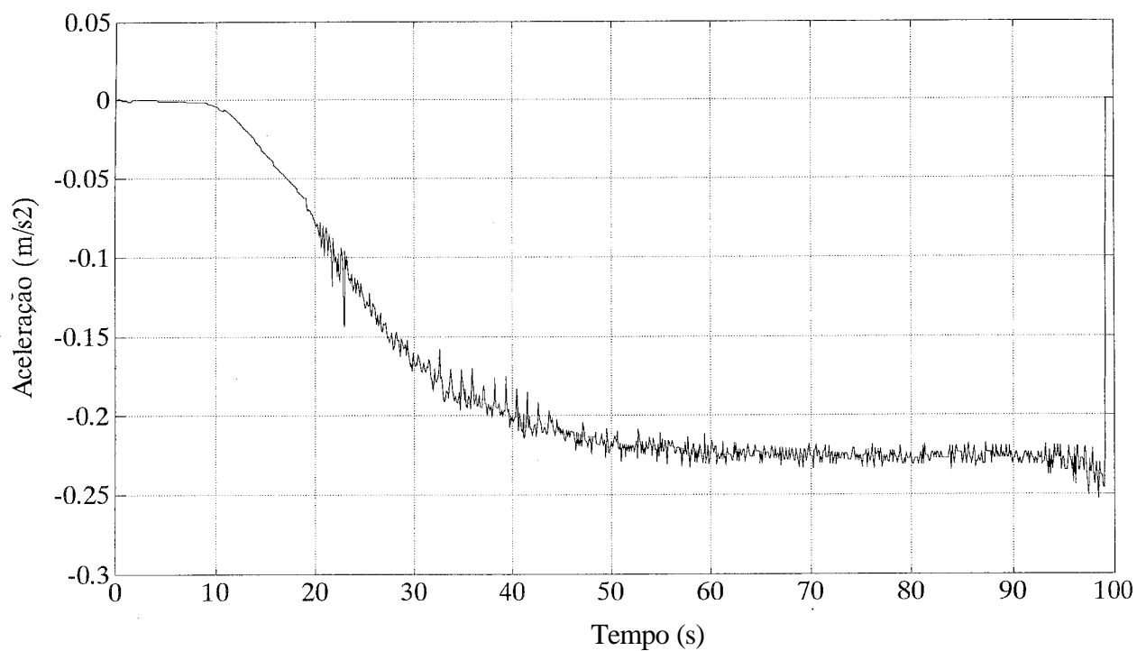
GRÁFICO 5 – Registro da Aceleração (1° Veículo)
