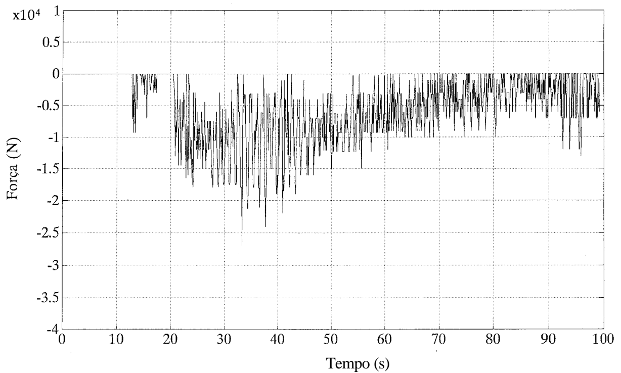
GRÁFICO 9 – Registro das Forças (13º Acoplamento)
