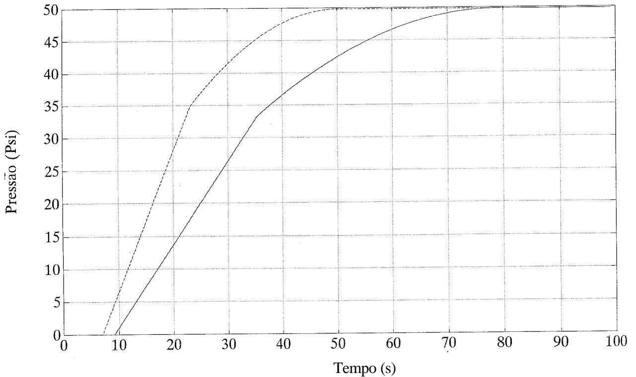
GRÁFICO 11 – Pressão do Cilindro de Freio (1º e 2º Veículos)
