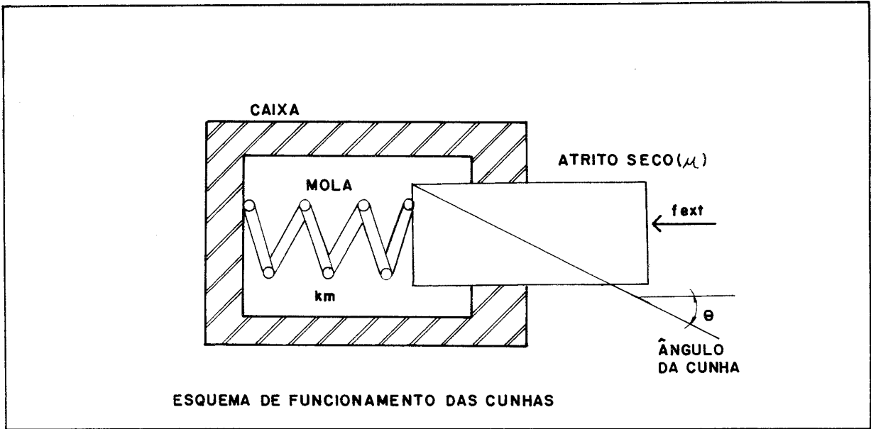
FIGURA 7 - Esquema das Cunhas do ACT
