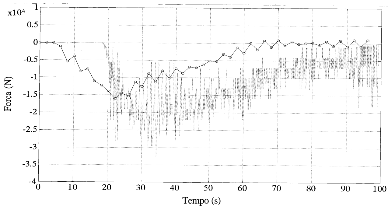
GRÁFICO 19 – Comparação das Forças (3 G.L.)
