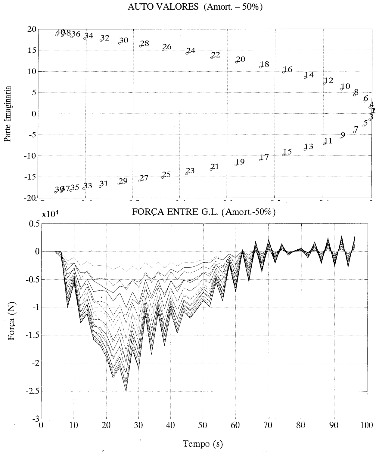
GRÁFICO D.5 - Amortecimento Minorado em 50%.
