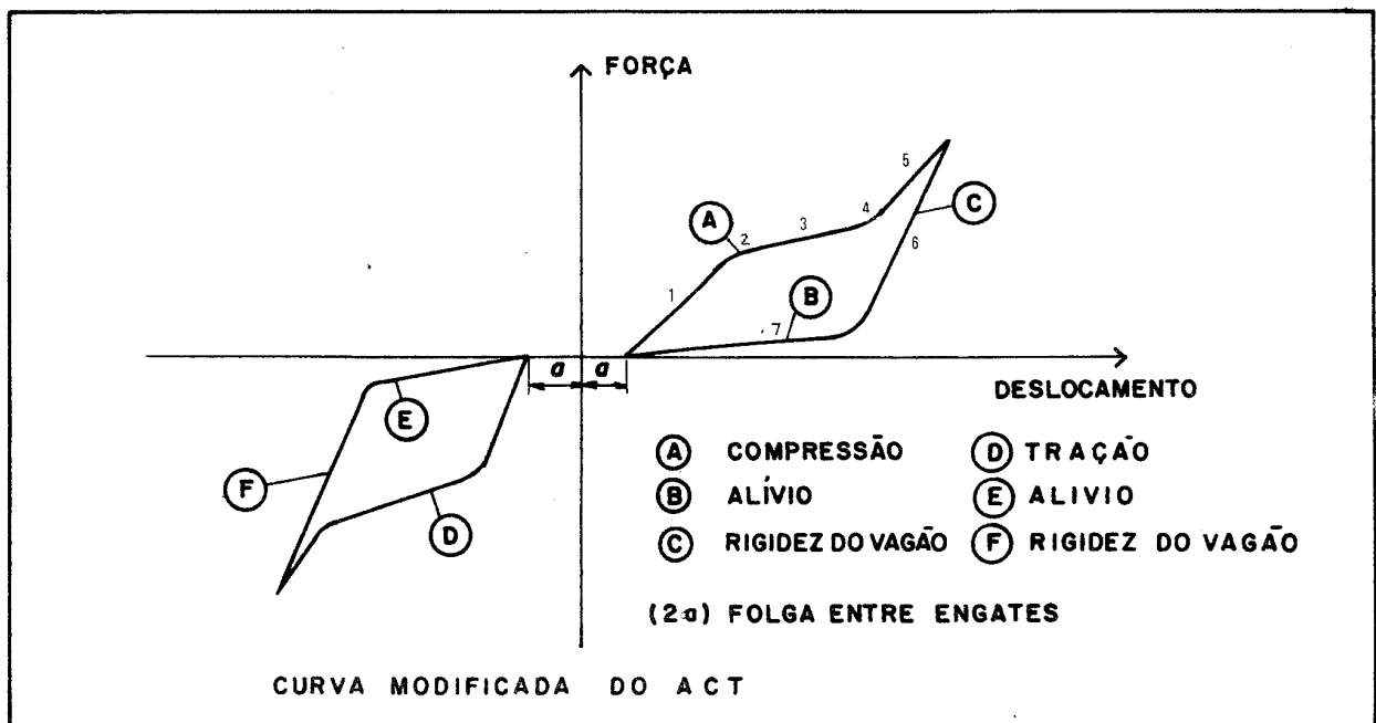
FIGURA A.4 – Curva do ACT
