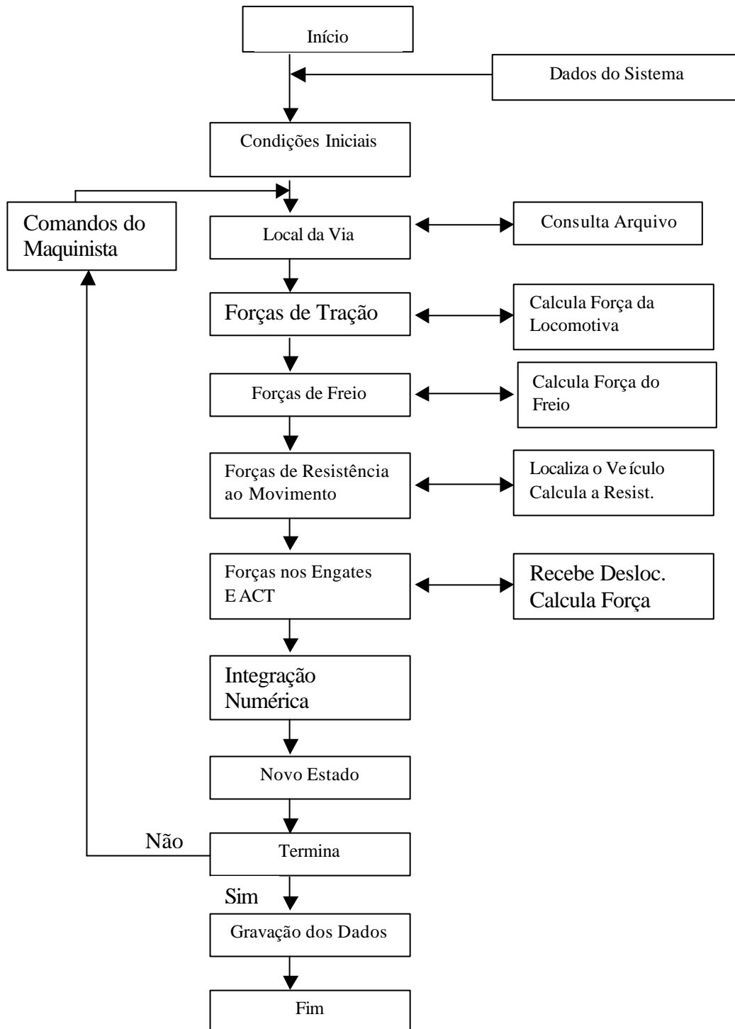
FIGURA 15 –Diagrama de Bloco do Programa
